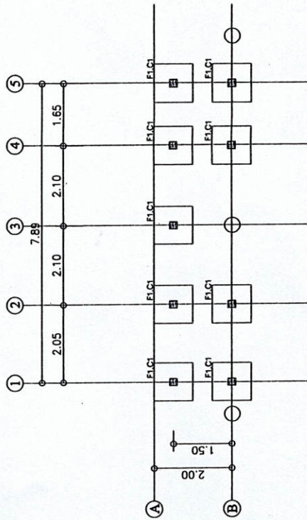
แบบแปลนงานฐานราก ขนาดตัวคน 1 : 100
